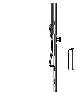
Vergrendeling 1490
