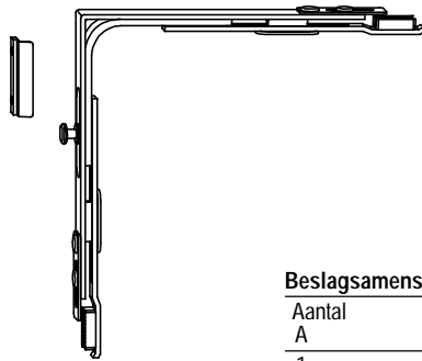
Hoekoverbrenging 6-32021-00-0-1 Sluitplaat volgens profiel
